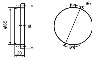
Рис.1. Габаритные и установочные размеры
